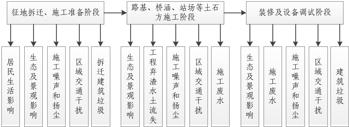
图 2.3-1 施工期工艺流程及产污环节示意图
