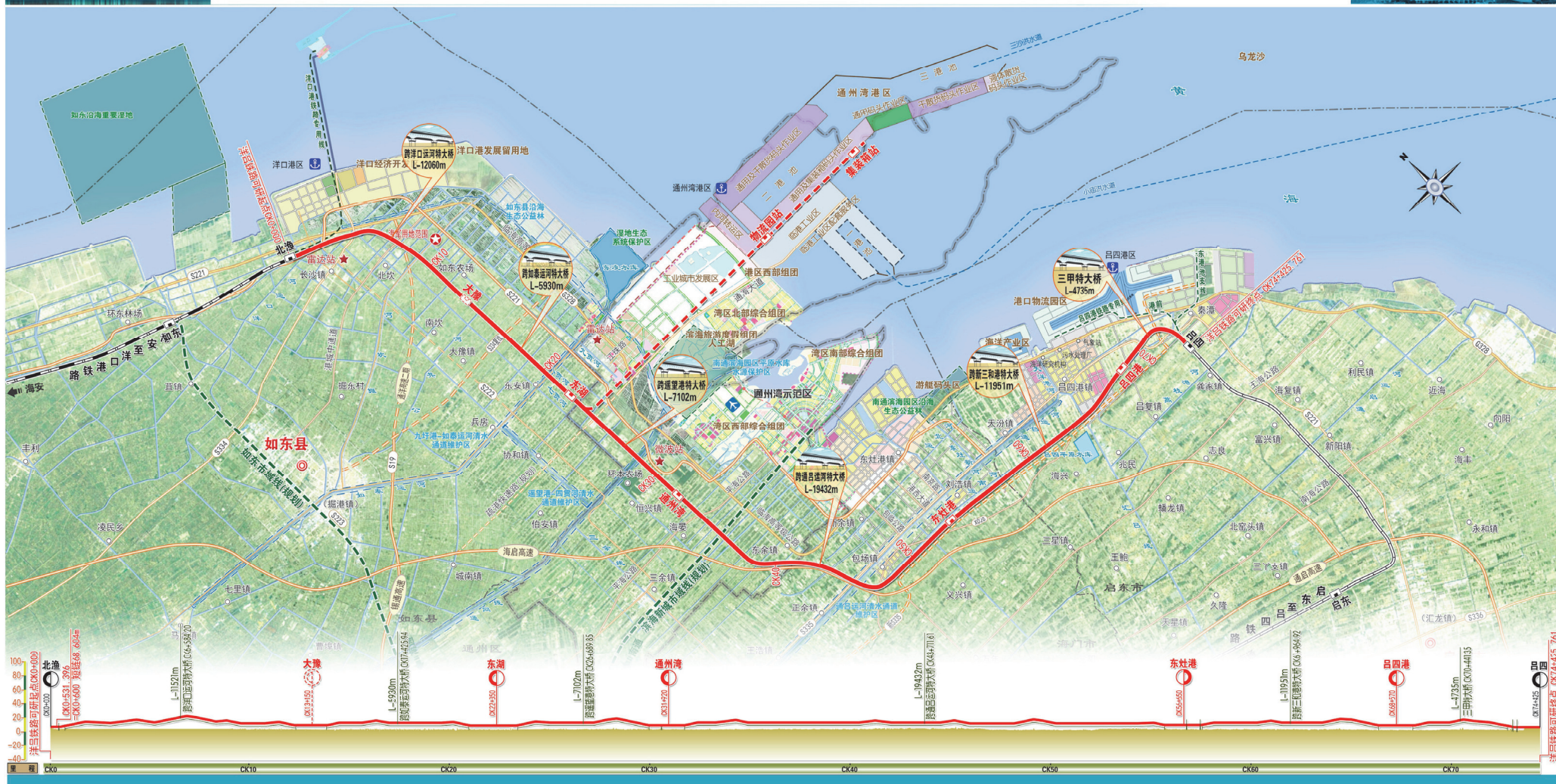
南通港洋口港区至吕四港区铁路联络线工程平纵断面示意图
